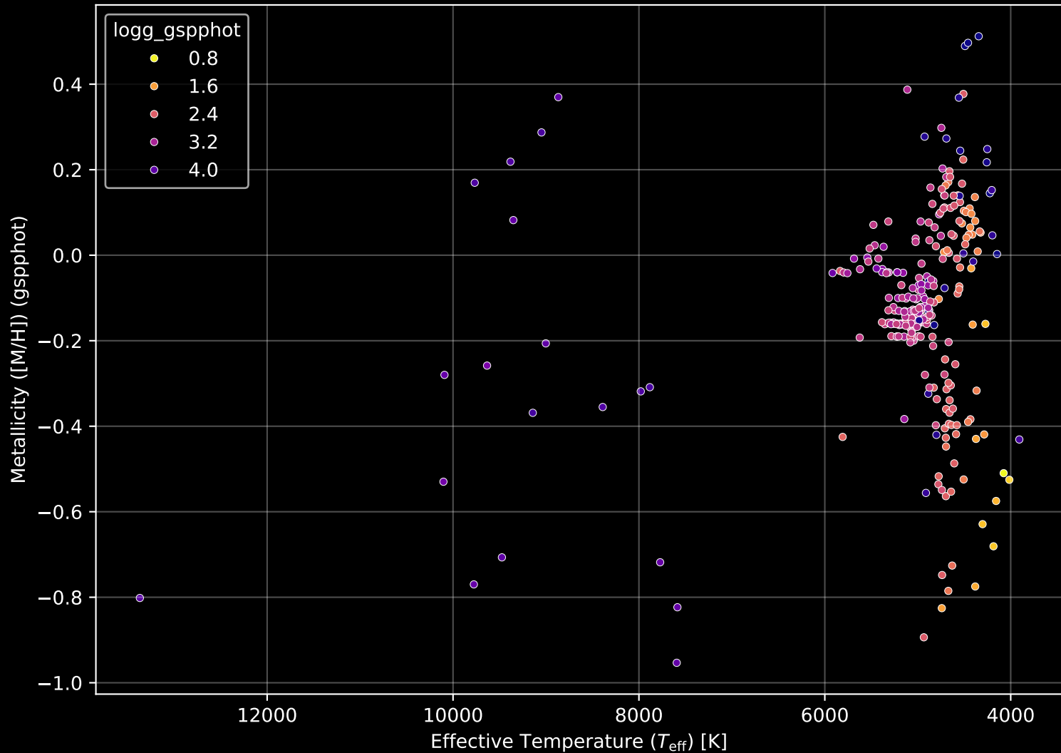
APOGEE DR17 Field: [169+12] Stellar Population Parameters (n= 299)
